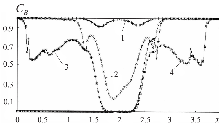
Рис. 6. Распределение концентраций бора C_B(x, y) в кремнии и диоксиде кремния вдоль оси x при различных значениях y = 0.20 (кривая 1), 0.61 (2), 1.0 (3) и 1.47 (4) для трехмасочной технологии отжига
