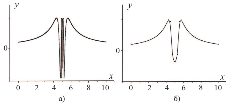
Рис. 7. График одной и той же функции F(x) = \sin \frac{1}{|x-5|} , отрисованный графической системой Origin с использованием дискретной сетки в 500 узлов (а) и 50 узлов (б)
