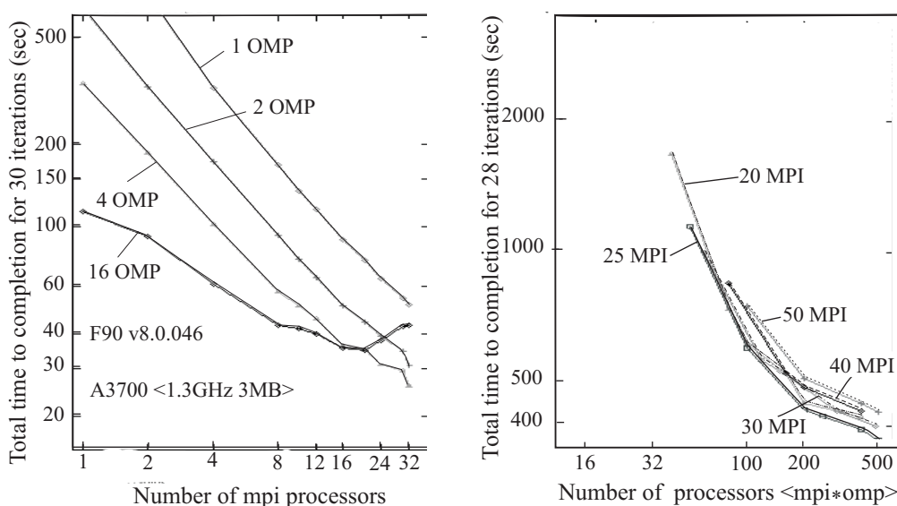
Рис. 4. Время, необходимое для выполнения 30 шагов полной модели с разрешением 0,9 \times 0,72 градуса (слева) и 28 шагов модели с разрешением 0,225 \times 0,18 градуса (справа), 28 вертикальных уровней на вычислительной системе Altix 3700 при различном сочетании числа процессоров MPI и OpenMP
