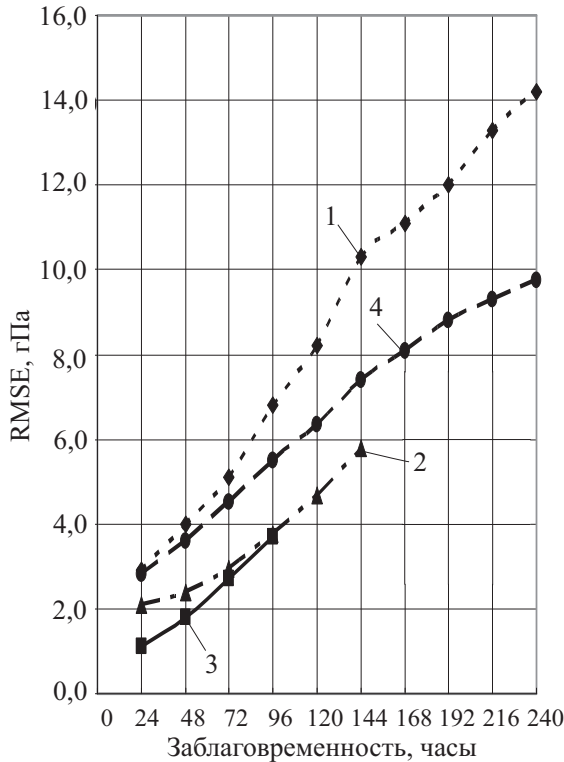
Рис. 6. График изменения осредненной среднеквадратической ошибки прогноза P_0 (давления на уровне моря) в зависимости от заблаговременности. Исходный срок 12 UTC. Регион: Северное полушарие. Период 2006 г. Оценка по сетке точек OA\ 2,5 \times 2,5^\circ SMA (1), RED (2), EXE (3), PL-AV (4)
