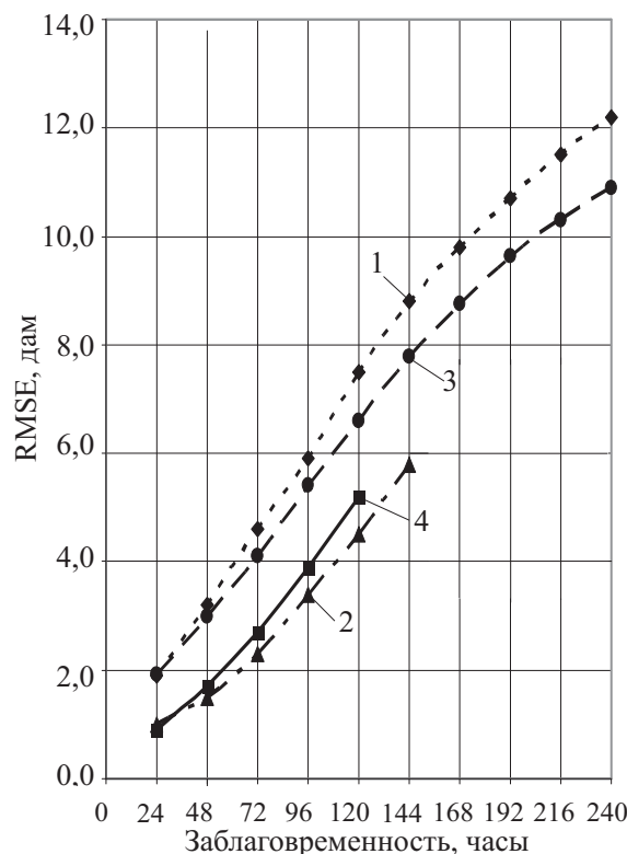
Рис. 5. График изменения осредненной среднеквадратической ошибки прогноза высоты поверхности 500 ГПа в зависимости от заблаговременности. Исходный срок 12 UTC. Регион: Северное полушарие. Период 2006 г. Оценка по сетке точек OA\ 2,5 \times 2,5^\circ . SMA (1), RED (2), PL-AV (3), EXE (4)
