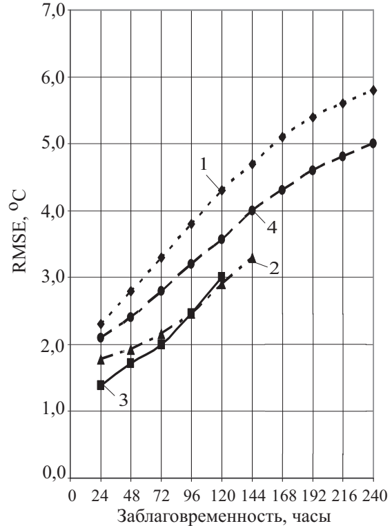
Рис. 7. График изменения осредненной среднеквадратической ошибки прогноза температуры на уровне 850 ГПа в зависимости от заблаговременности. Исходный срок 12 UTC. Регион: Северное полушарие. Период 2006 г. Оценка по сетке точек OA\ 2,5 \times 2,5^\circ . SMA (1), RED (2), EXE (3), PL-AV (4)
