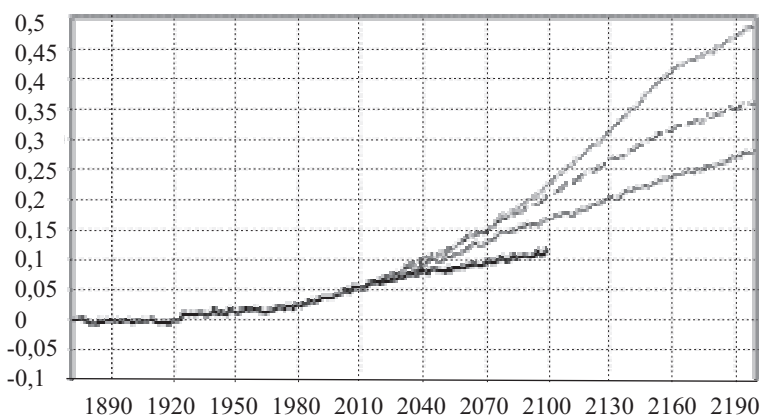
Рис. 3. Изменение уровня моря (м) в экспериментах XX и XXI (сплошная жирная линия), B1 (тонкая линия), A1B (штриховая линия) и A2 (пунктирная линия) по отношению к контрольному эксперименту
