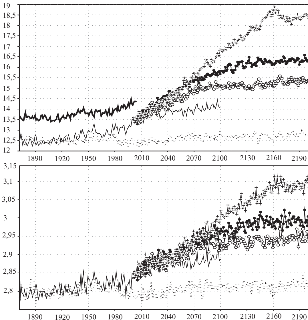
Рис. 1. Изменение интегральной температуры приземного воздуха в градусах Цельсия (вверху) и осадков в мм/сут (внизу) в контрольном эксперименте (пунктирная жирная линия), экспериментах XX и XXI (сплошная тонкая линия), B1 (открытые кружки \circ ), A1B (черные кружки \bullet ) и A2 (крестики + ). Сплошной жирной линией показано наблюдаемое изменение температуры
