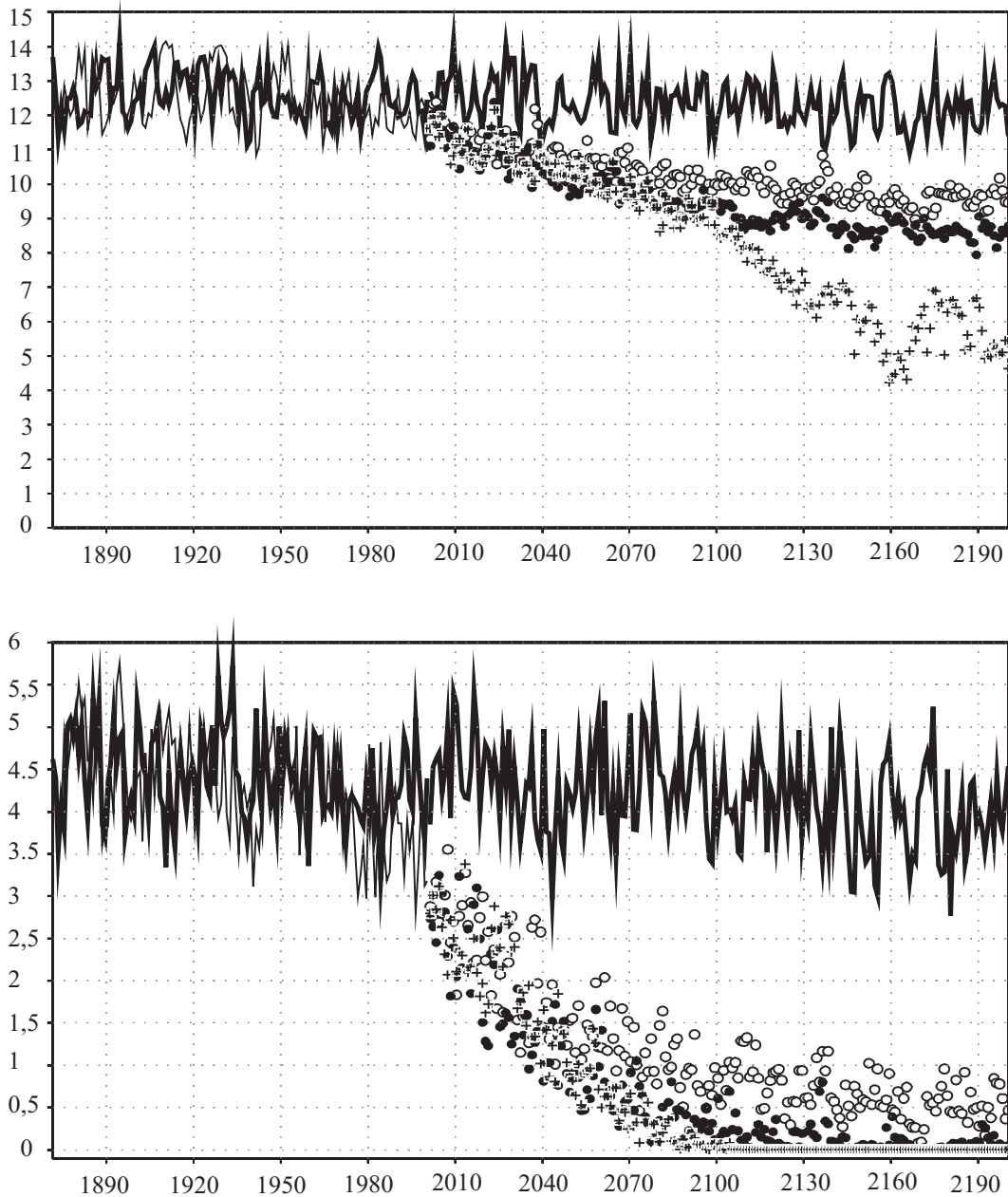
Рис. 2. Площадь морского льда в северном полушарии в млн кв. км в марте (вверху) и сентябре (внизу) по данным контрольного эксперимента (жирная линия), эксперимента XX (тонкая линия), экспериментов B1 (открытые кружки ○), A1B (черные кружки ●), A2 (крестики +)
